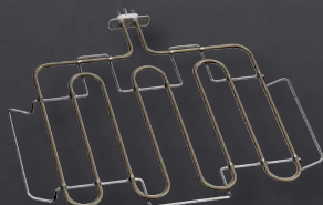
BA 056 113 Heizkörper für Backstein und Gastronorm-Bräter
